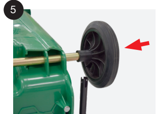
5 Insertamos una de las ruedas (B1) hasta que oigamos un clic, y seguidamente hacemos lo mismo con la otra rueda (B2).
