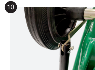
10 Insertamos el clip retenedor (F) según imagen.
