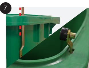
7 Con la tapa abierta, localizamos unas incisiones en el contenedor, e insertamos las guías verticales eleva-tapas (D) como se muestra en la imagen.
